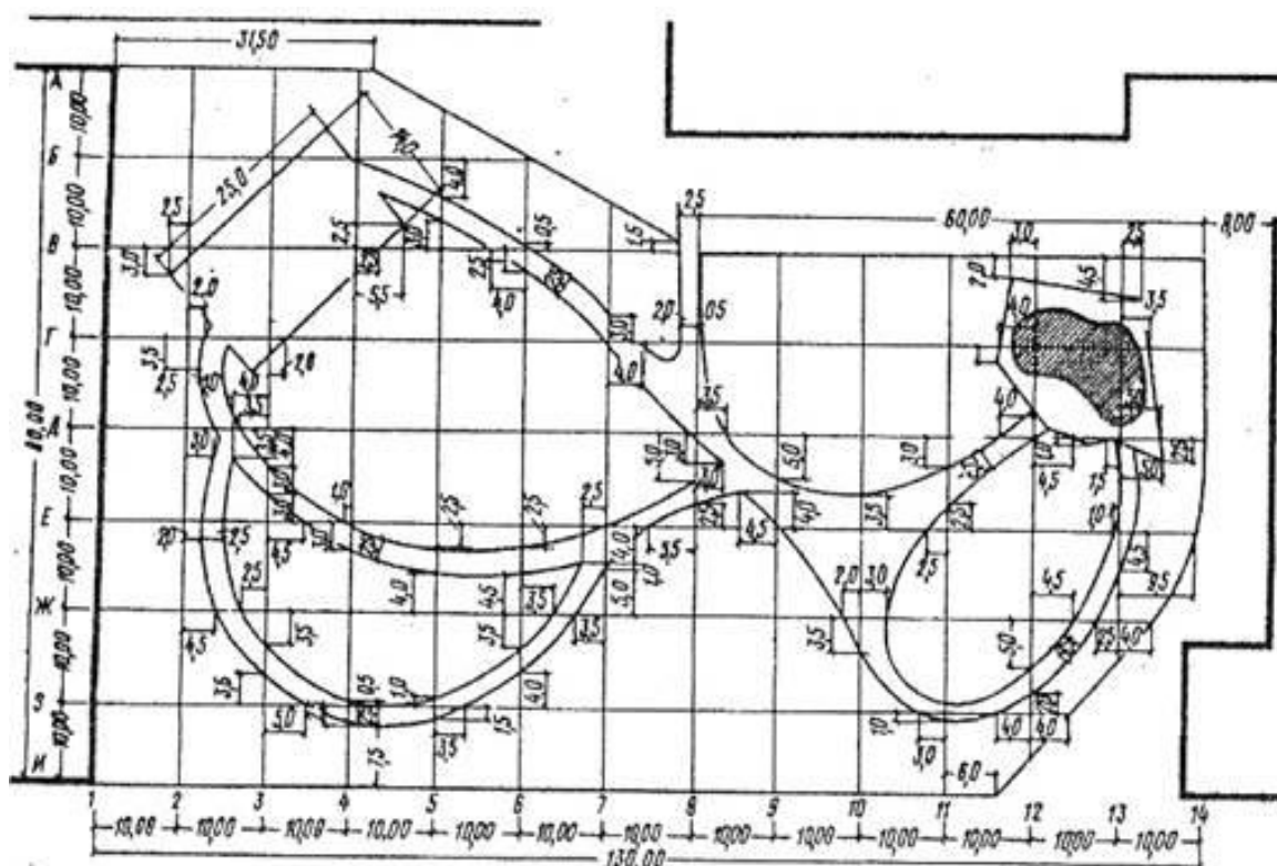
Рис. 4. Приклад виконання розбивочного креслення ПЕРЕЛІК ВИКОРИСТАНИХ ЛІТЕРАТУРНИХ ДЖЕРЕЛ
